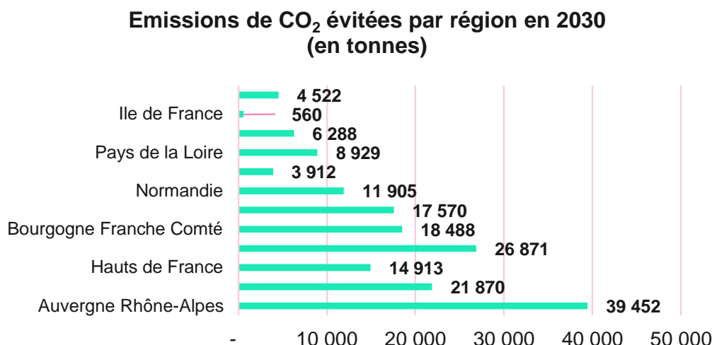
FIGURE 18 : REPARTITION REGIONALE DES REDUCTIONS D'EMISSIONS DE CO 2
