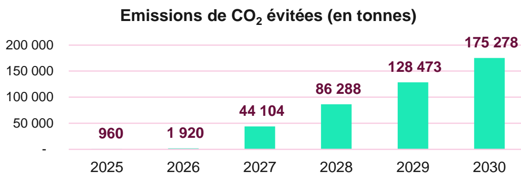
FIGURE 17 : TRAJECTOIRE DE REDUCTIONS DES EMISSIONS DE CO 2 POUR LE SCENARIO INTERMEDIAIRE
