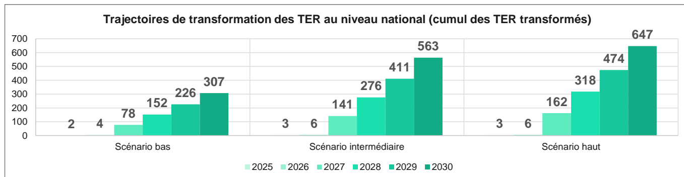
FIGURE 1 : EVOLUTION DU MATERIEL ROULANT AU BIOGNV JUSQU'À 2030 (CUMUL DES TER TRANSFORMES) 3
