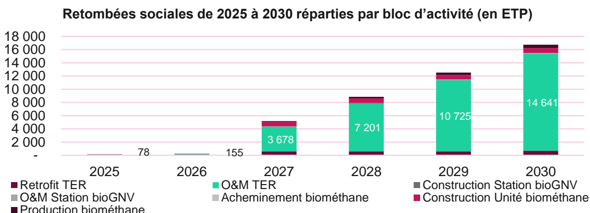
FIGURE 5 : ESTIMATION DES EMPLOIS GENERES SUR LES DIFFERENTS SEGMENTS D'ACTIVITE
